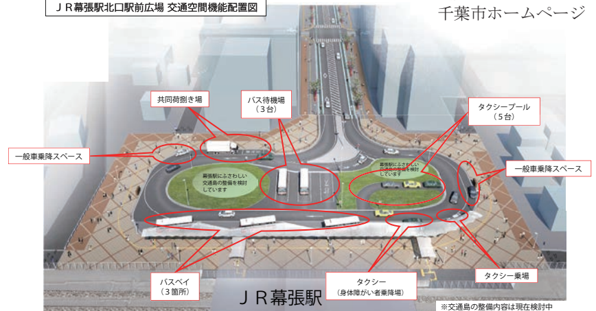
JR幕張駅北口駅前広場 交通空間機能配置図
